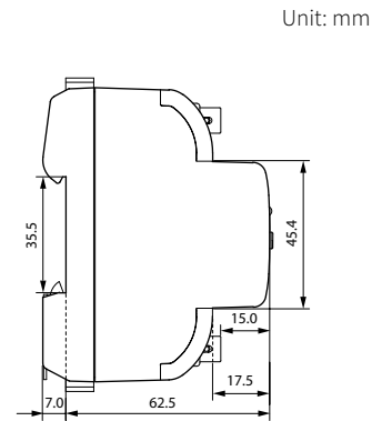
Dimensions
